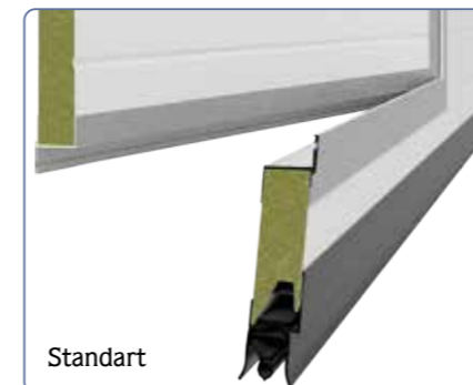
Standart ve Düşük Eşikli Servis Kapısı Detayları
